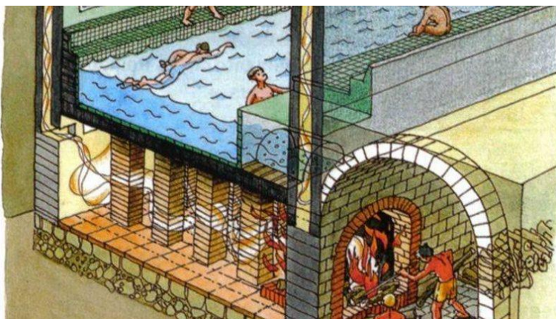
* Slika 8: Rimski hipokavst I Slika 9: Rimsko kopališče
